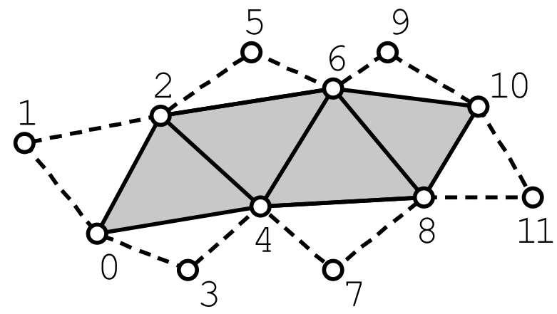
GL_TRIANGLE_STRIP_ADJACENCY
