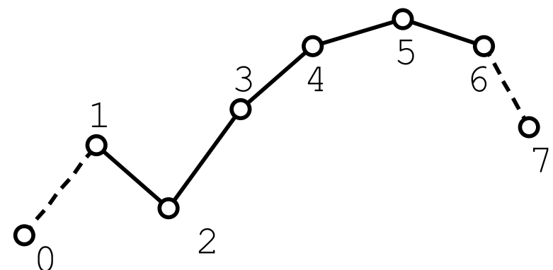
GL_LINE_STRIP_ADJACENCY
